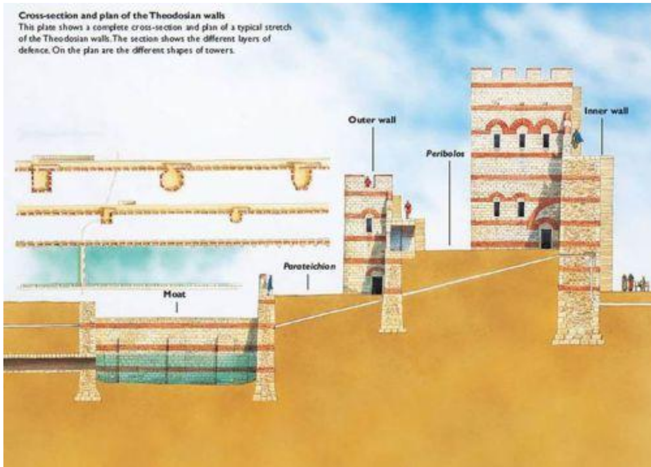
Sección de las murallas con torres y fosos
