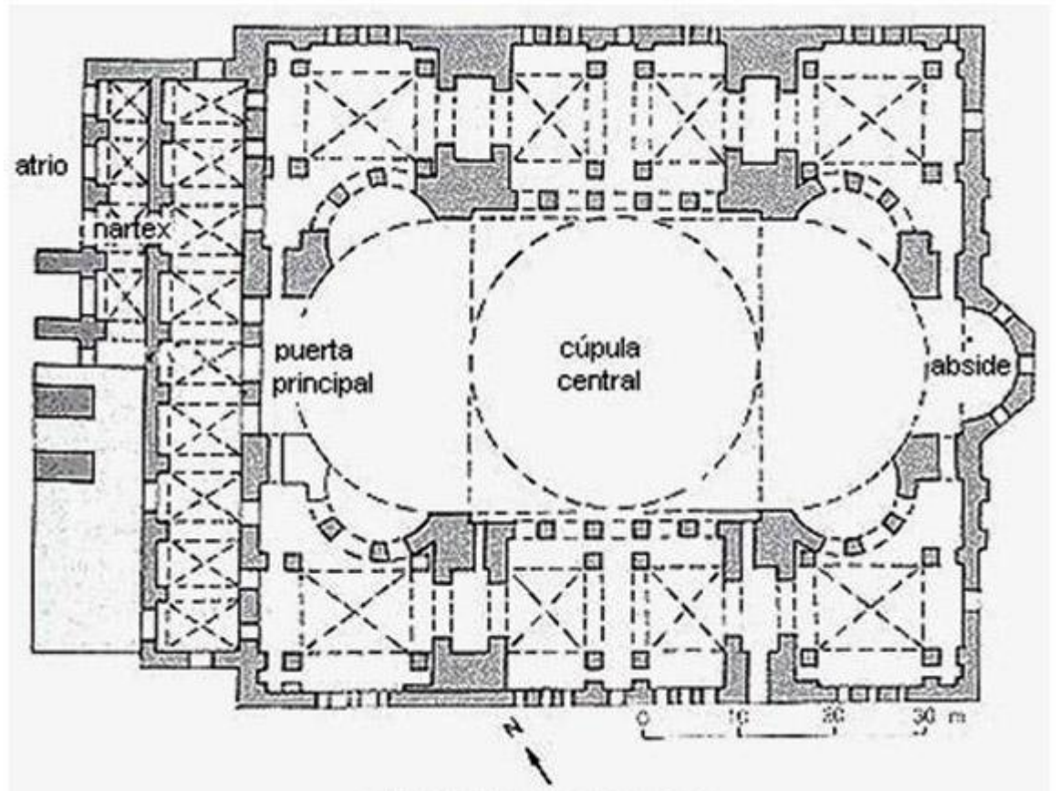
Santa Sofía o Hagia Sophía , planta
